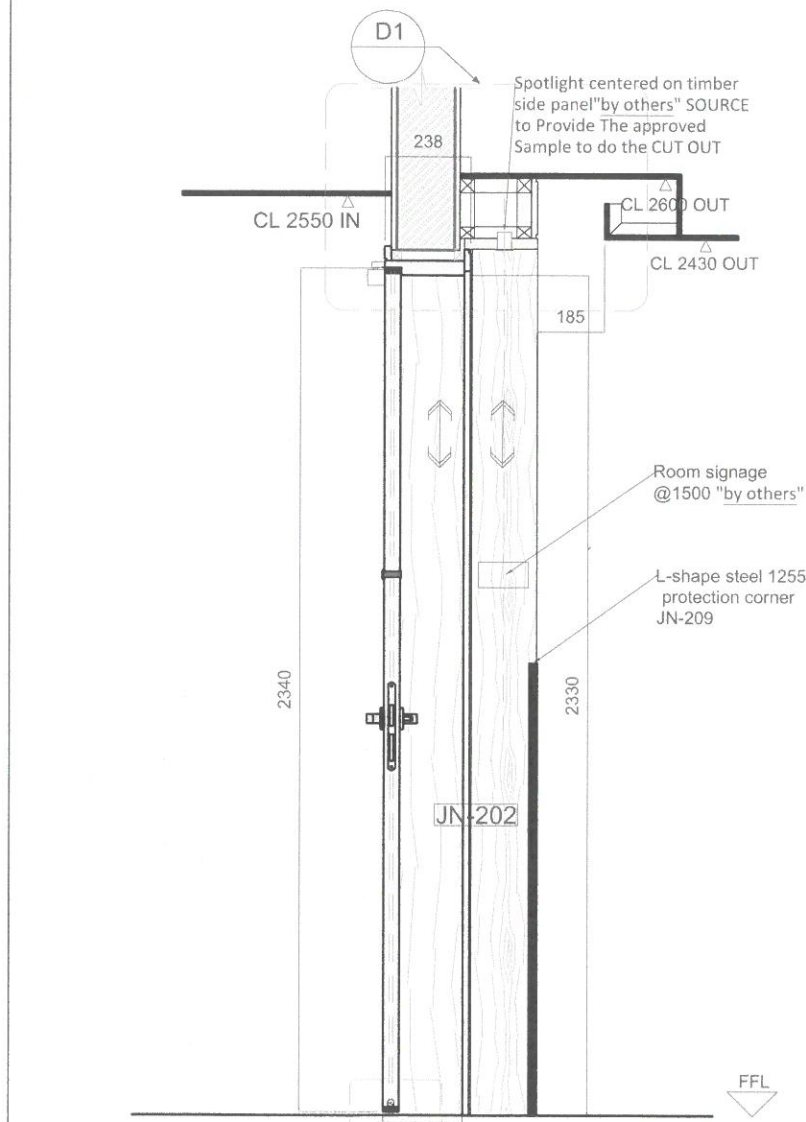
D2 SC1 Section
